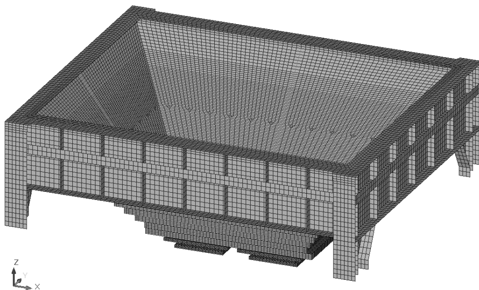
Рис. 2. СЕМ бункеру агломерату комбінату «Криворіжсталь»
